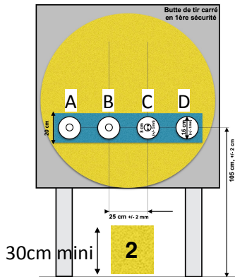
Cible papier \varnothing 16 \text{ cm} \pm 1 \text{ mn} 4 cibles Cordons 1 mn à l'avantage
