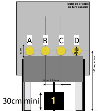
Cible à bascule \varnothing 16 \text{ cm} \pm 1 \text{ mn} 4 cibles
